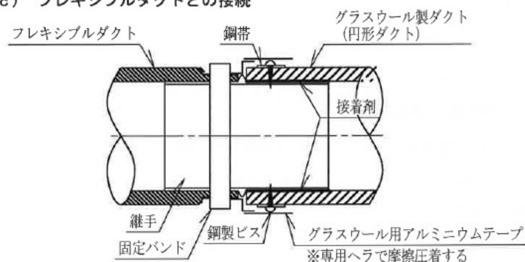
（c） フレキシブルダクトとの接続
